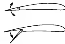
Закрилок
